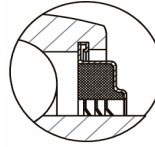
Vedação R3
